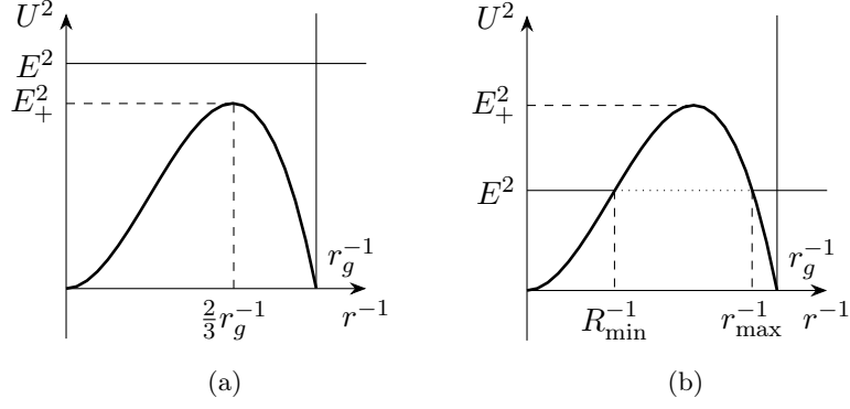
Рис. 12.2. Случай нулевой массы: (а) E > E_+ ; (б) E < E_+ .
